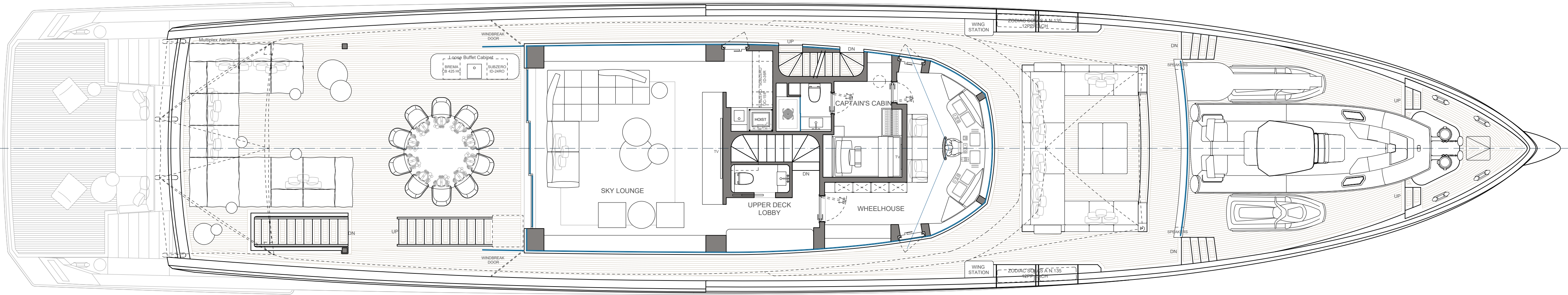
-5 0 5 10 15 20 25 30 35 40 45 50 55 60 65 70 UPPER DECK
