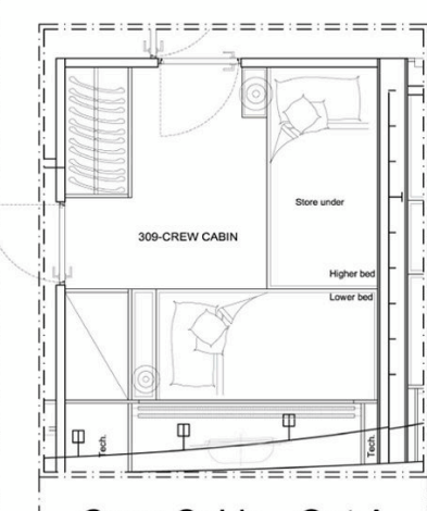
Crew Cabin - Opt.A
